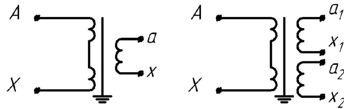
Рисунок 2 - Принципиальная электрическая схема и маркировка выводов трансформаторов напряжения НОЛ-СЭЩ-6(10)-IV-2 с одной и двумя вторичными обмотками.
