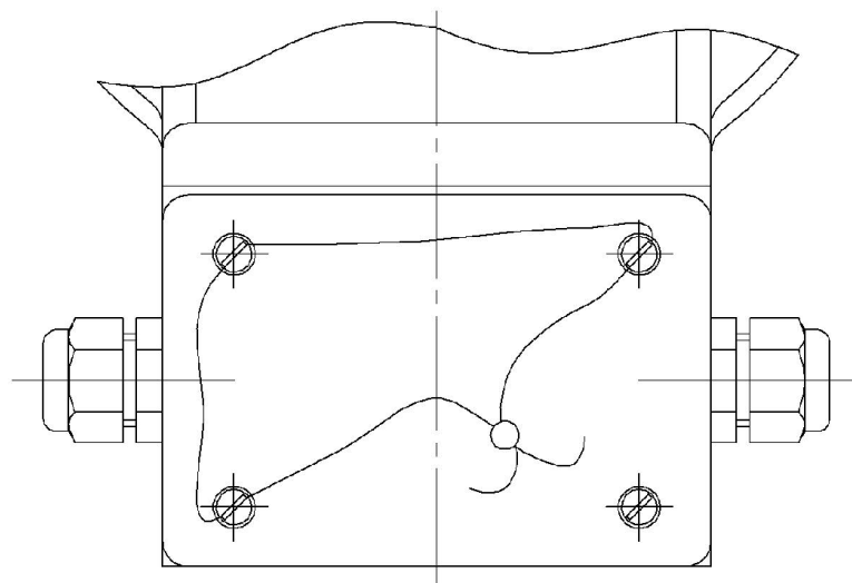
Рисунок 3 - Рекомендуемая схема пломбировки вторичных выводов трансформаторов НОЛ-СЭЩ-6(10)-IV-2
