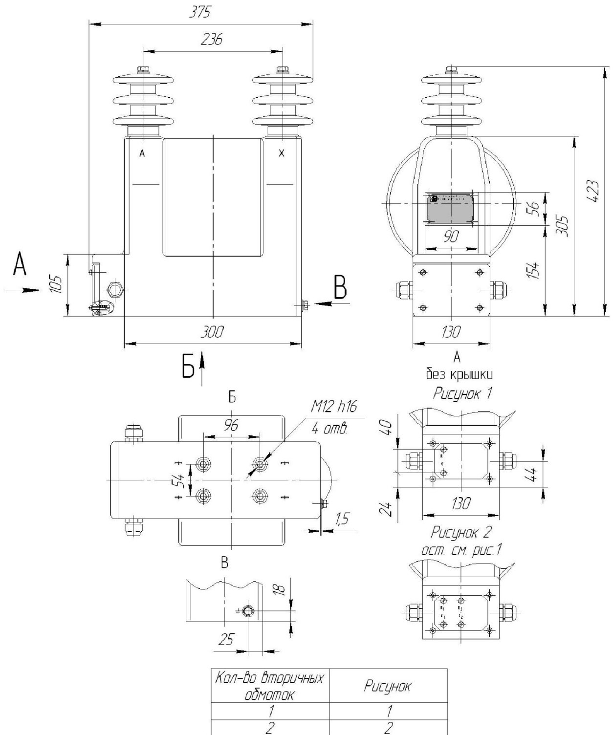
Рисунок 1 - Габаритные, установочные и присоединительные размеры трансформаторов напряжения НОЛ-СЭЩ-6(10)-IV-2
