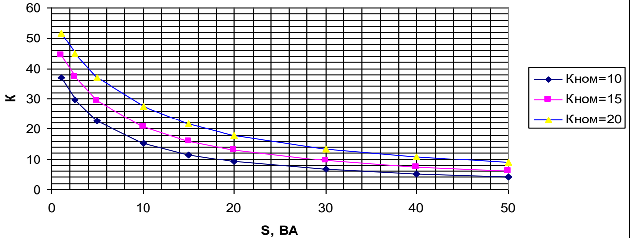
Кривые предельной кратности вторичных обмоток для защиты с классами точности 5P и 10P и номинальной нагрузкой 15 ВА трансформаторов с первичным током 1000А
