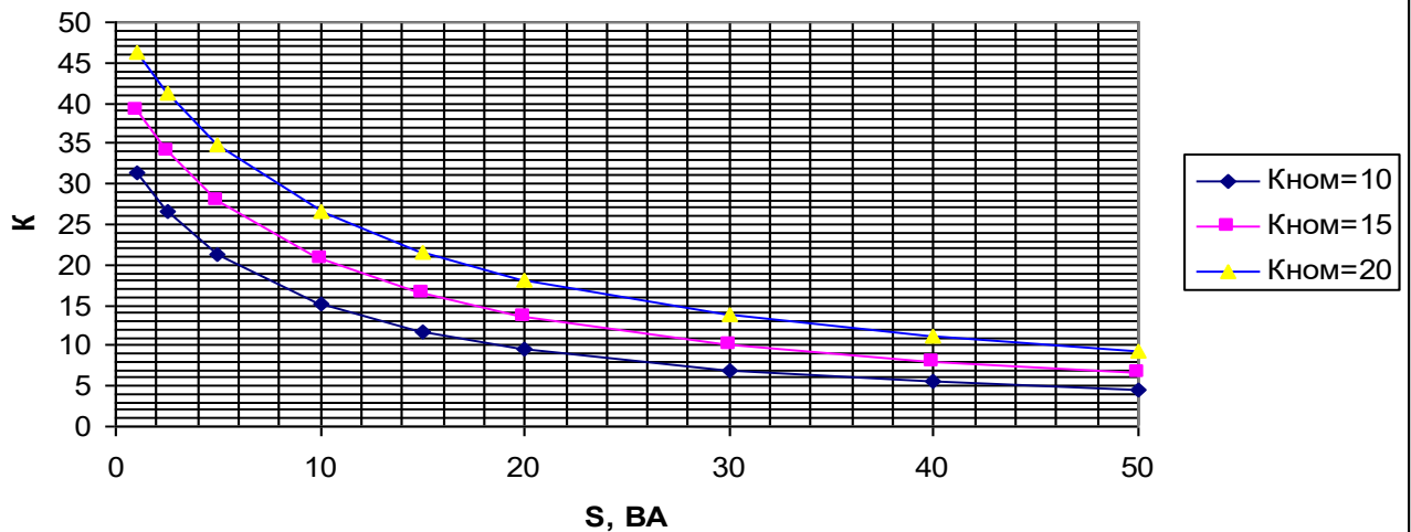
Кривые предельной кратности вторичных обмоток для защиты с классами точности 5P и 10P и номинальной нагрузкой 15 ВА трансформаторов с первичным током 1500А
