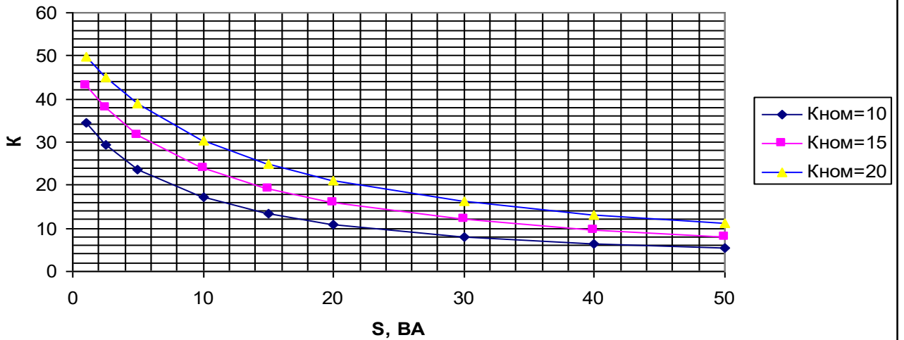
Кривые предельной кратности вторичных обмоток для защиты с классами точности 5P и 10P и номинальной нагрузкой 20 ВА трансформаторов с первичным током 1500А
