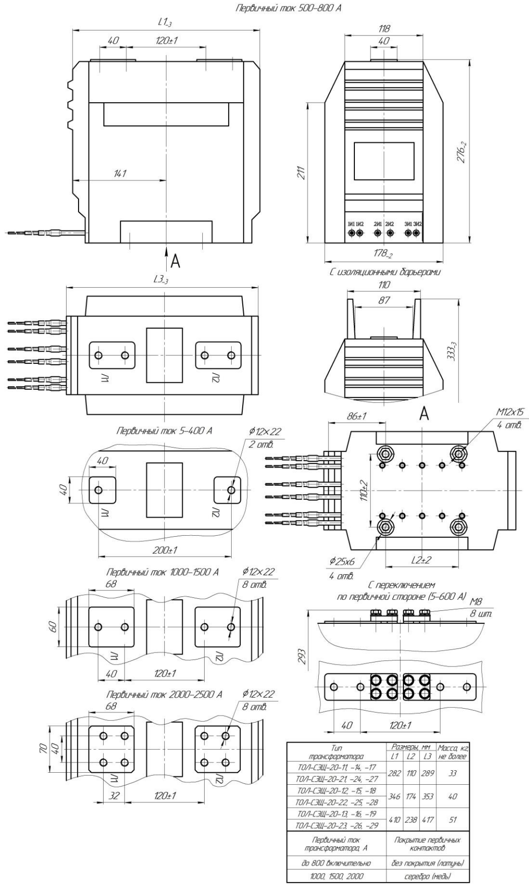
Рисунок 3 Габаритные, установочные и присоединительные размеры трансформаторов тока ТОЛ-СЭЦ-20 исполнений 11÷19, 21÷29 с гибкими выводами
