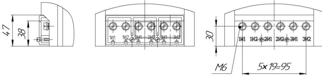
Рисунок 5 Расположение вторичных выводов трансформаторов тока ТОЛ-СЭЦ-10 исполнений 11÷19, 21÷29
