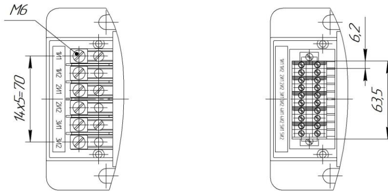
Рисунок 4 Расположение вторичных выводов трансформаторов тока ТОЛ-СЭЦ-10 исполнений 01÷09, 31÷39
