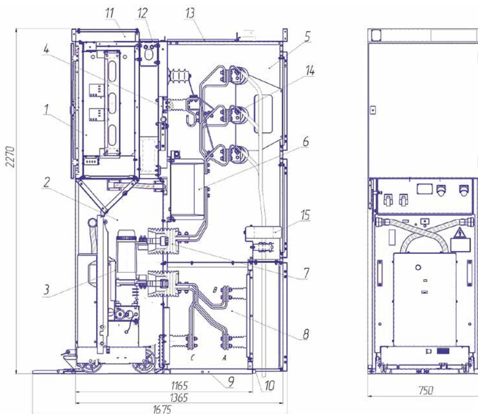
Рисунок 2. Шкаф кабельного ввода (вывода)
