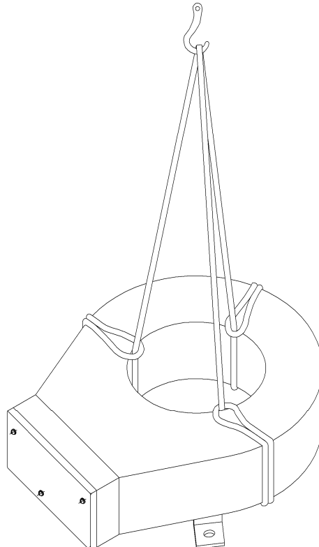
Рис. 2 – Схема строповки без упаковки
