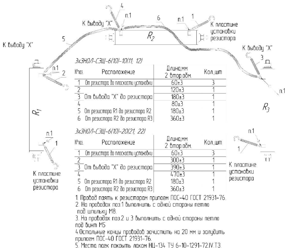
Рисунок 5 - Монтажная схема соединения резисторов
