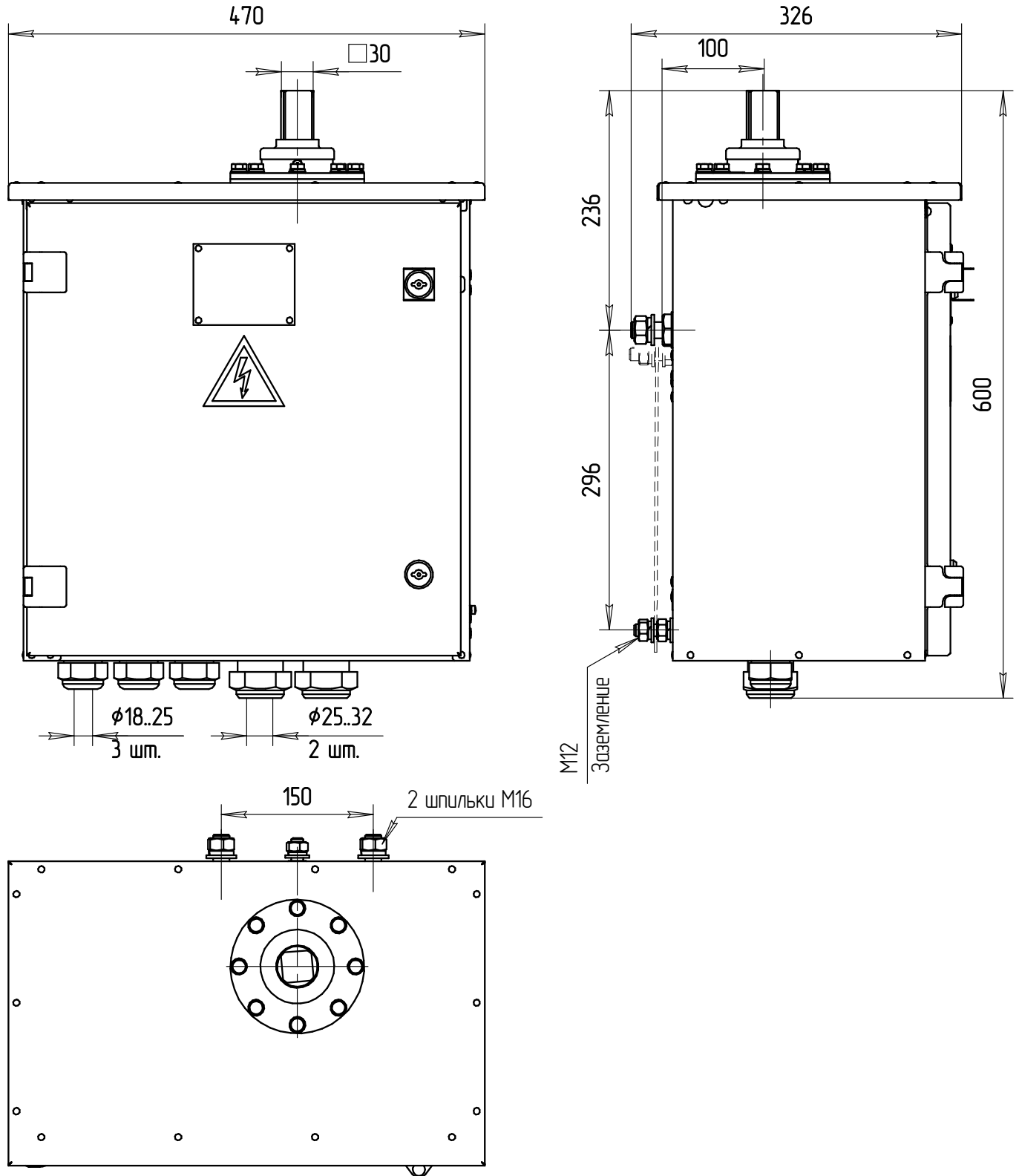
Рисунок А.1 – Общий вид привода ПД СЭЩ ® -11-190 УХЛ1
