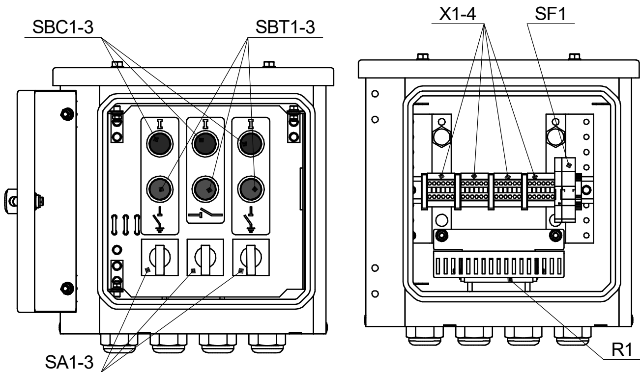
Рисунок А.3 – Расположение элементов выносного блока управления ВБУ
