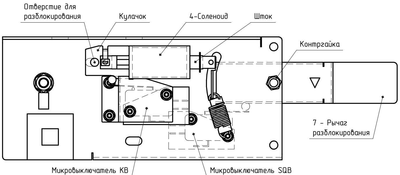
Рисунок В.2 – Конструкция механизма ручного оперирования - вид изнутри
