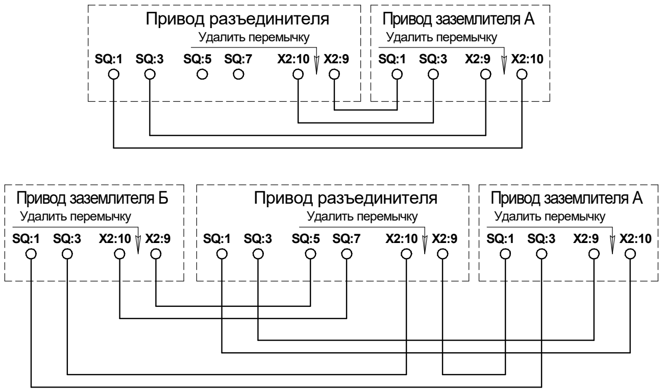
Рисунок Б.6 – Схема организации электрической блокировки между приводом главных ножей разъединителя и приводами заземлителей (пример)
