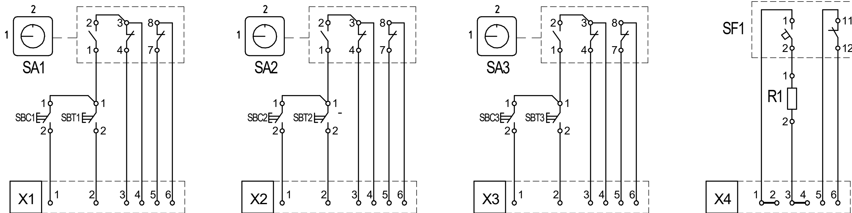
Схема электрическая принципиальная выносного блока управления ВБУ-1.3
