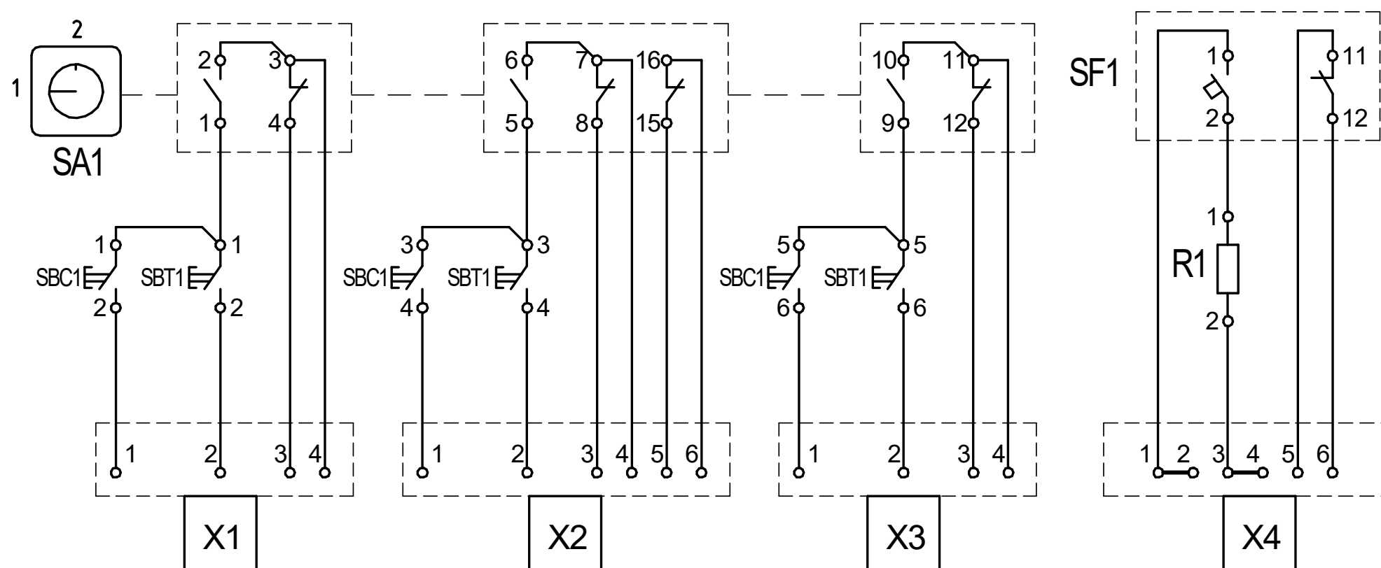
Схема электрическая принципиальная выносного блока управления ВБУ-31 (для группового управления тремя разъединителями)
