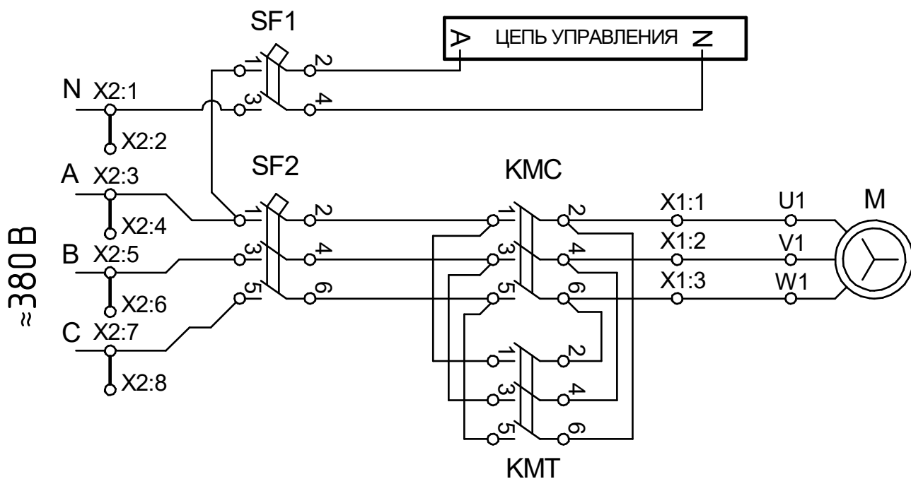
Рисунок Б.1 – Силовые цепи привода ПД СЭЩ®-11-190 UXЛ1
