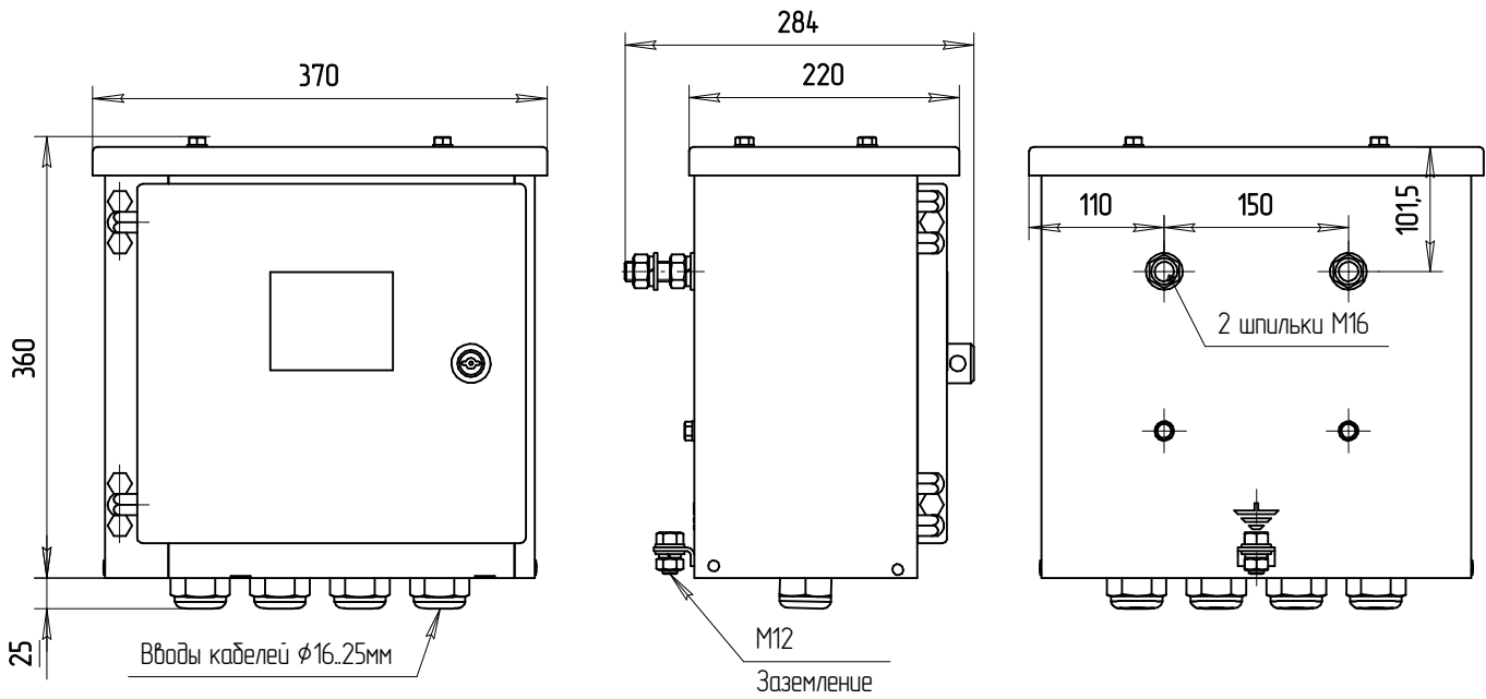
Рисунок А.2 – Выносной блок управления ВБУ
