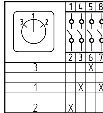
Диаграмма работы переключателя SA
