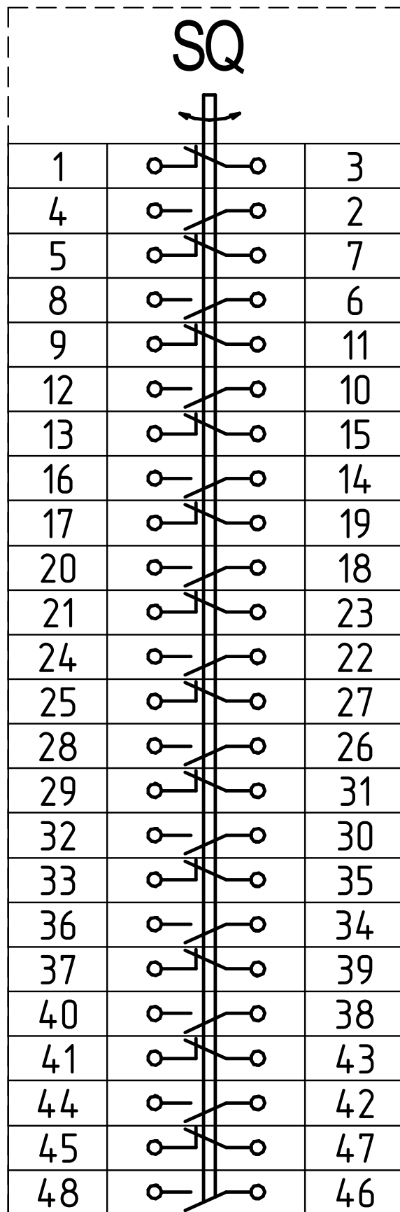
Рисунок Б.3 – Цепи вспомогательных контактов блокировки и сигнализации состояния SQ привода ПД СЭЩ ® -11-190 УХЛ1
