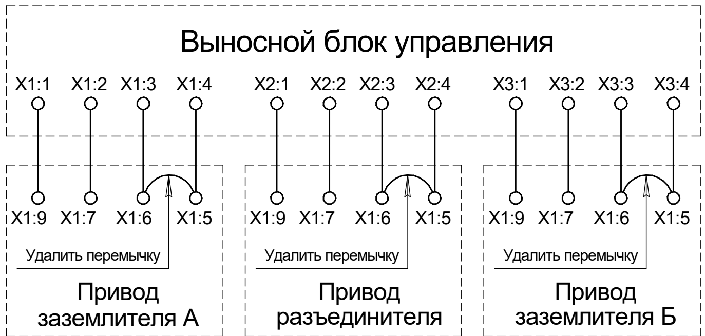
Рисунок Б.7 – Схема соединения выносного блока управления с приводами
