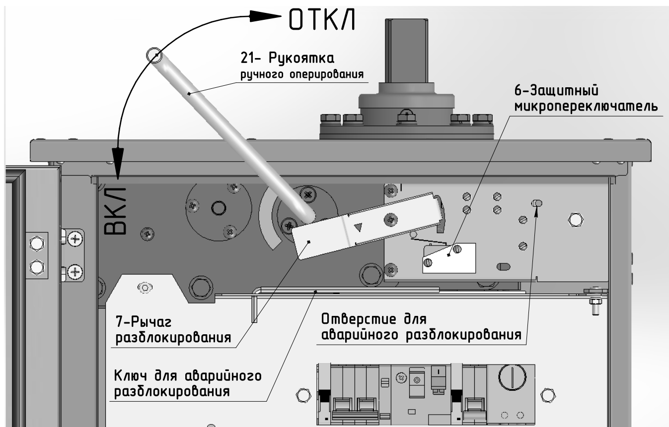
6–Микровыключатель SQB; 7–Рычаг разблокирования; 21–Рукоятка Рисунок 4 – Ручное оперирование
