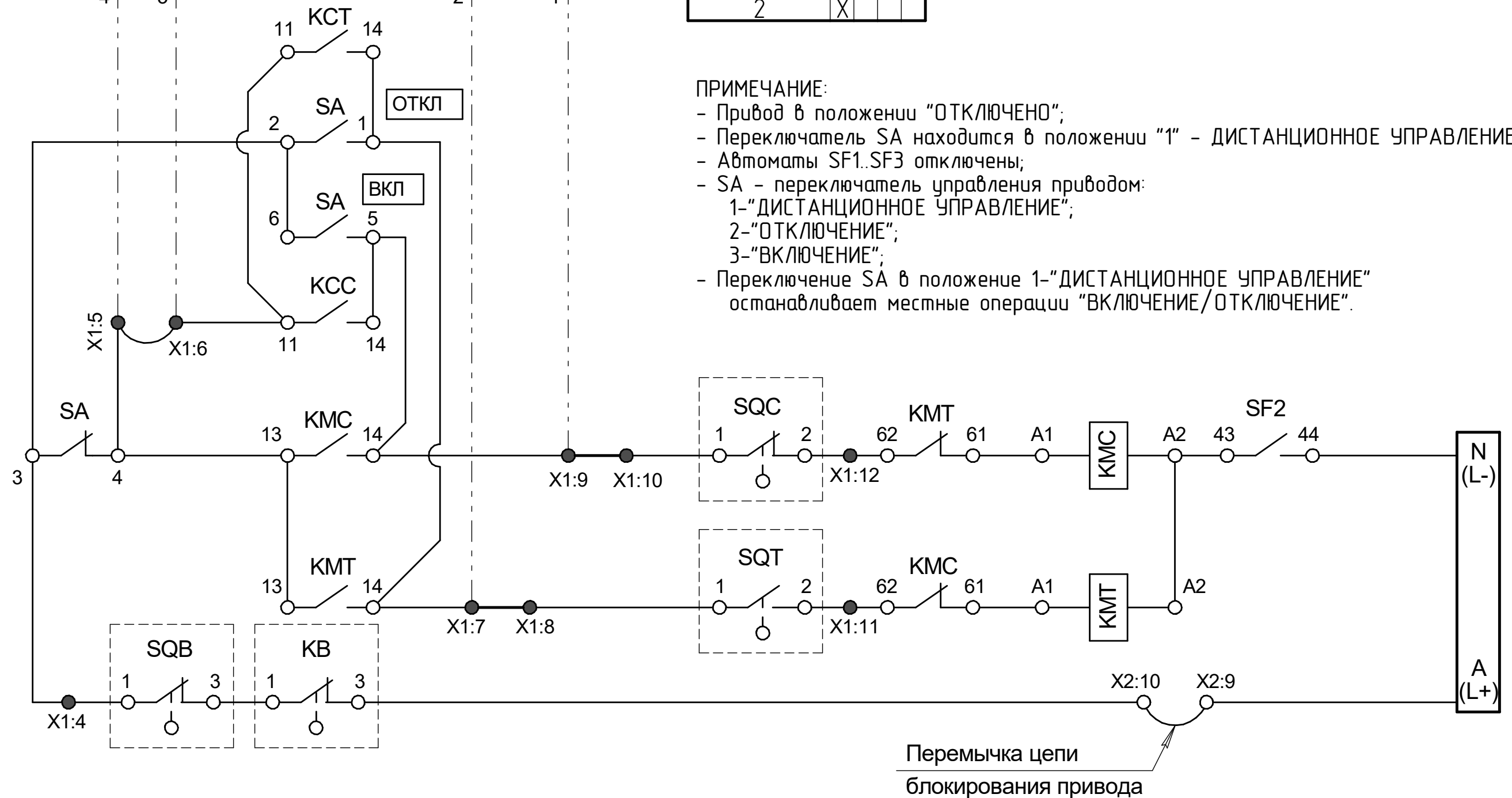
Рисунок Б.4 – Цепь управления привода ПД СЭЩ®-11-190 УХЛ1
