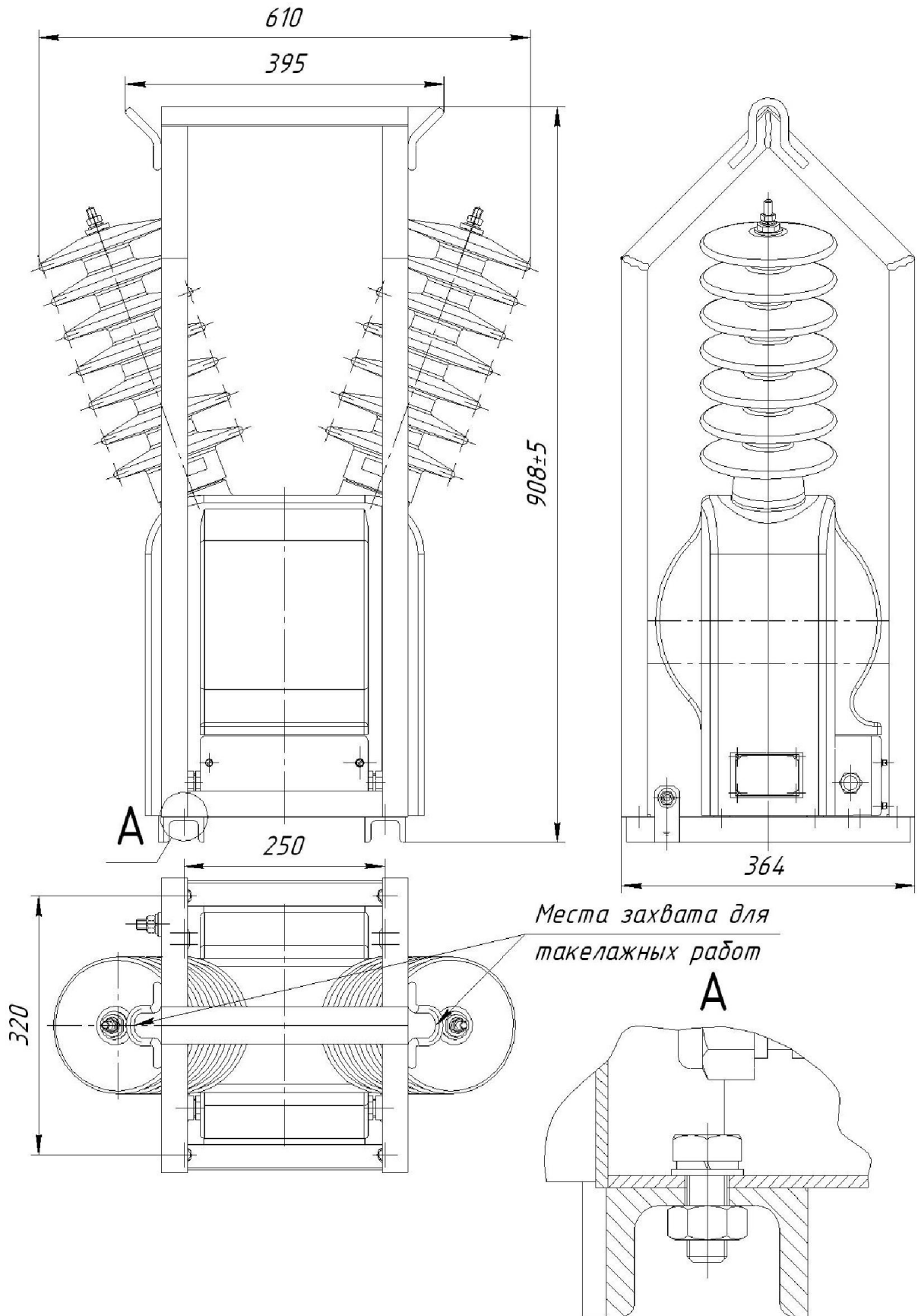
Рисунок 3 - Габаритные размеры трансформаторов напряжения НОЛ-СЭЩ-35-IV на транспортировочной раме.
