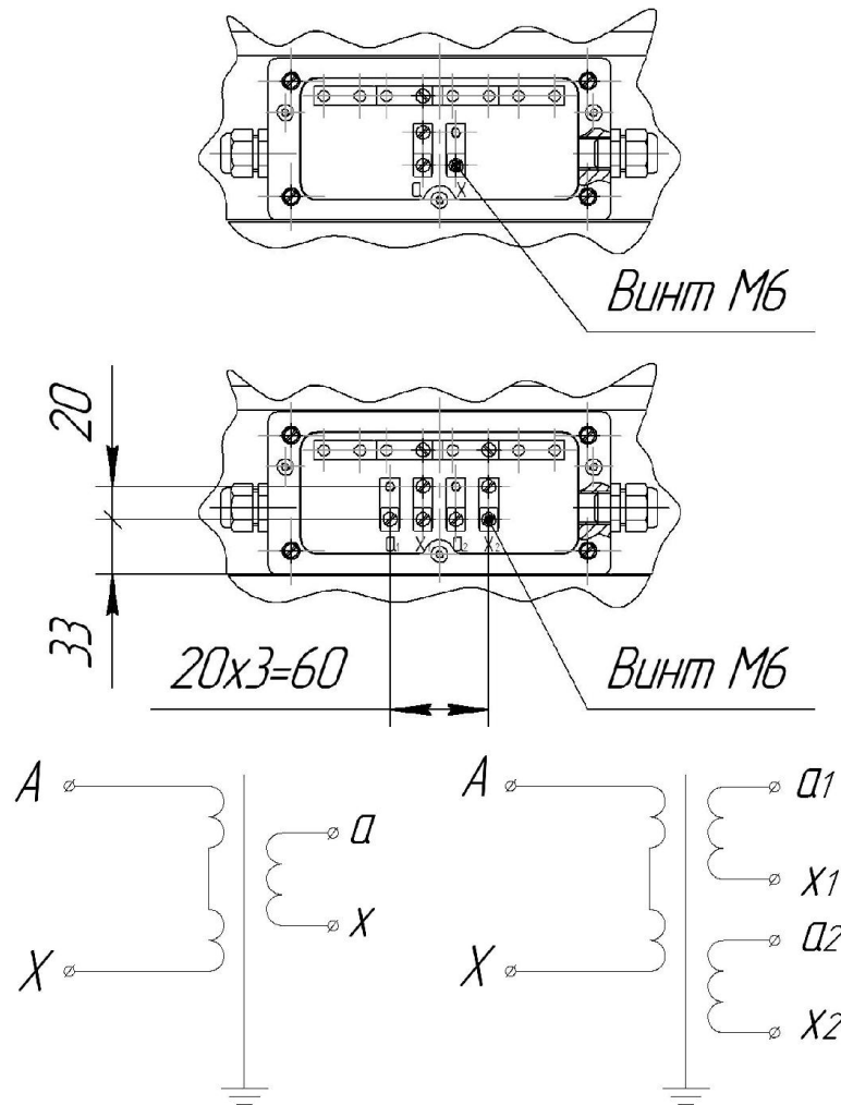
Рисунок 2 - Принципиальная электрическая схема и маркировка выводов трансформаторов напряжения НОЛ-СЭЦ-35-IV
