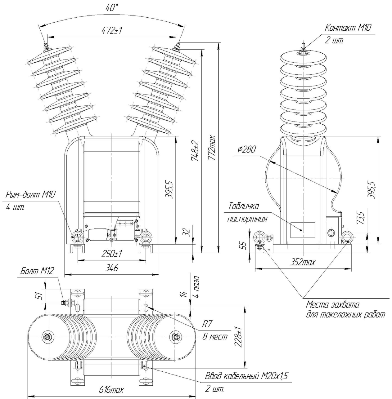
Рисунок 1 - Габаритные, установочные и присоединительные размеры трансформаторов напряжения НОЛ-СЭЦ-35-IV
