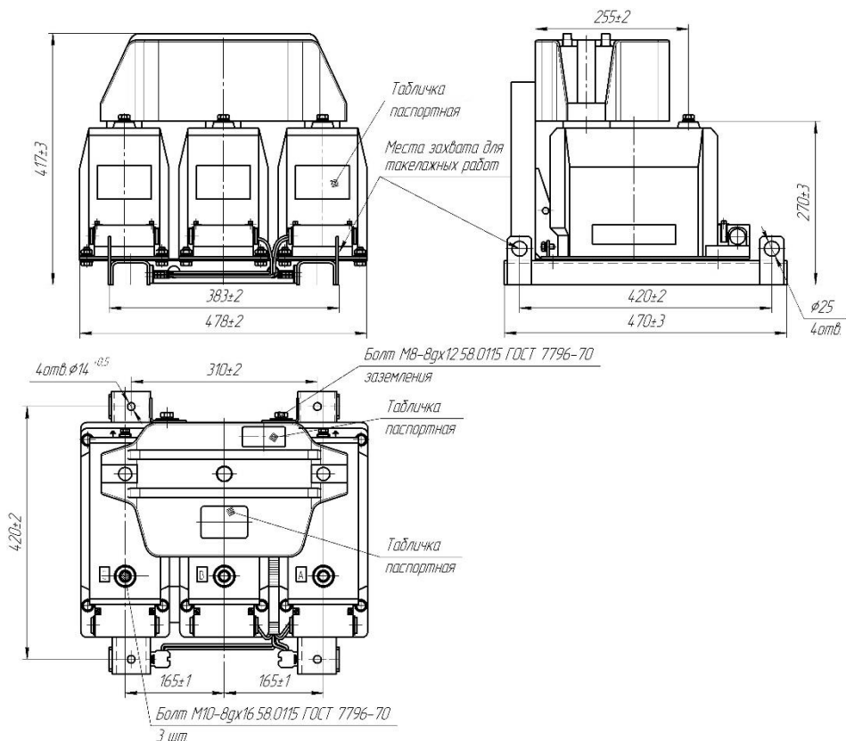
Рисунок 1 Габаритные, установочные, присоединительные размеры трехфазных групп НАЛИ-СЭЩ-6(10)-3
