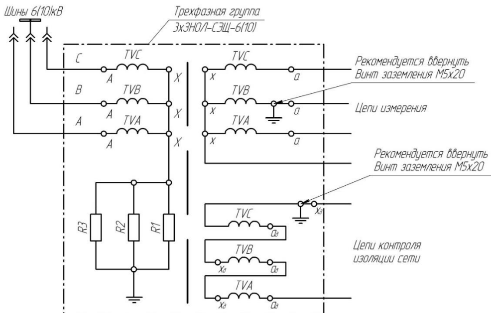
Рисунок 2 - Принципиальная электрическая схема соединения обмоток трехфазной группы измерительных трансформаторов 3xЗНОЛ-СЭЦ-6(10)-20 с двумя вторичными обмотками
