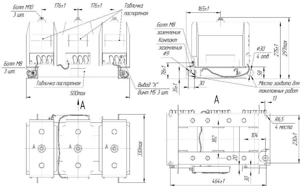
Рисунок 1 - Габаритные, установочные, присоединительные размеры и масса трехфазной группы измерительных трансформаторов 3хЗНОЛ-СЭЩ-6(10)-20
