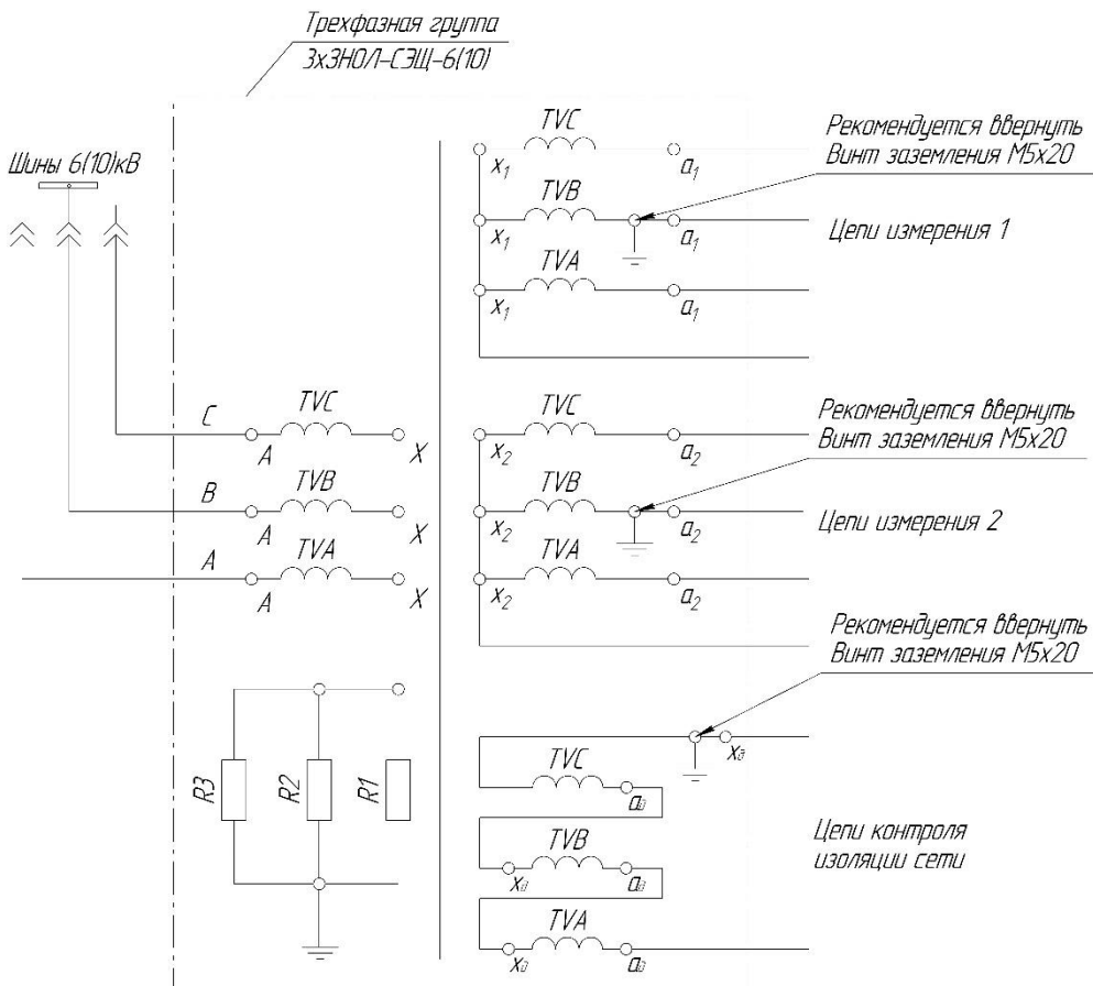
Рисунок 3 - Принципиальная электрическая схема соединения обмоток трехфазной группы измерительных трансформаторов 3хЗНОЛ-СЭЦ-6(10)-10 с тремя вторичными обмотками.
