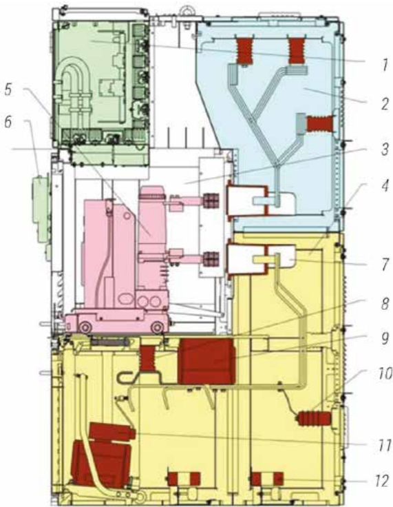
Классическая компоновка ячейки КРУ-СЭЩ-70 10 кВ
