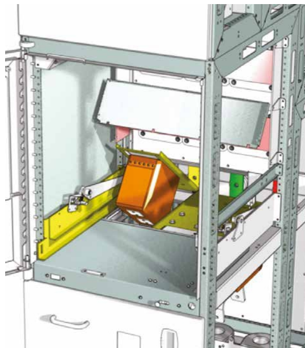
Демонтаж трансформаторов тока в КРУ-СЭЩ-70-10
