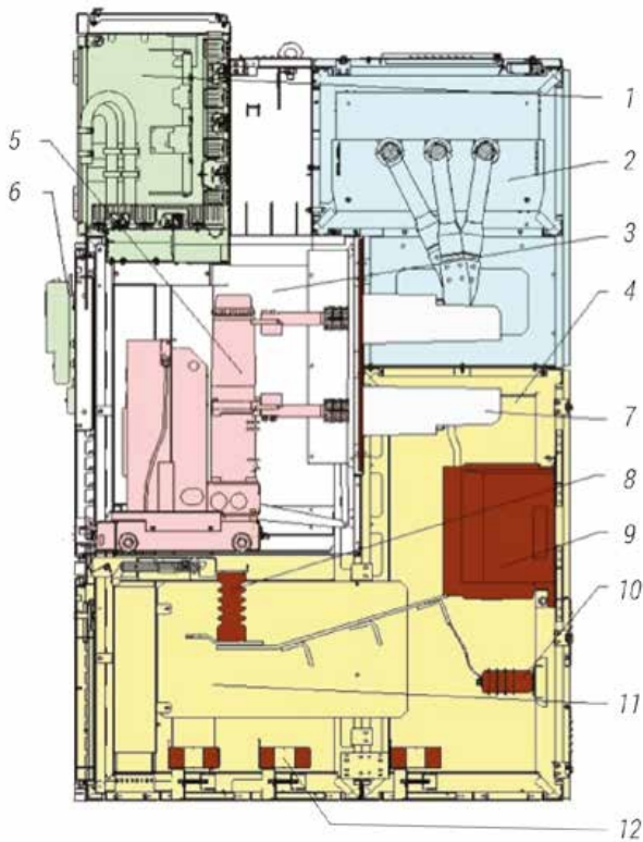
Классическая компоновка ячейки КРУ-СЭЩ-70 20 кВ
